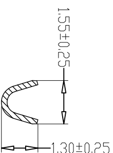
SEC:B-B
