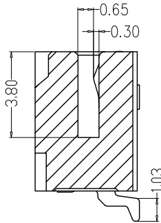
SEC.A-A
